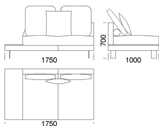
Siedzisko 1 z półką
