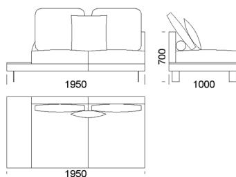
Siedzisko 2 z półką
