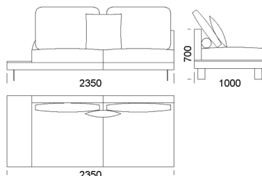
Siedzisko 4 z półką
